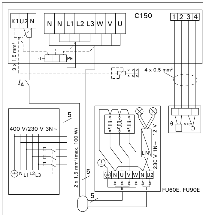
Рисунок 12а. Электромонтаж пульт управления C150 и каменки FU-E (подключение в 3-фазной сети)
