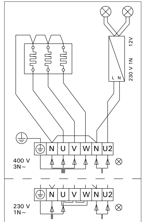
Рисунок 11. Подключение камней FU-E Joonis 11. Keriste FU-E elektrühendused
