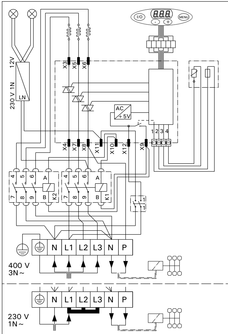
Рисунок 10. Подключение камней FU Joonis 10. Keriste FU elektrühendused
