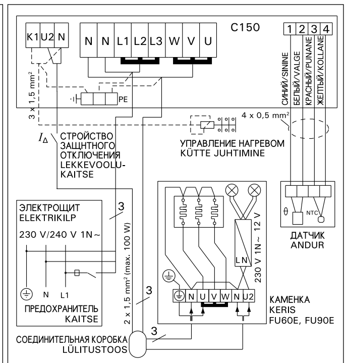
Рисунок 12б. Электромонтаж пульт управления C150 и каменки FU-E (подключение в 1-фазной сети)
